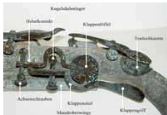
Klappe am Oberbügel innen, Detailansicht
